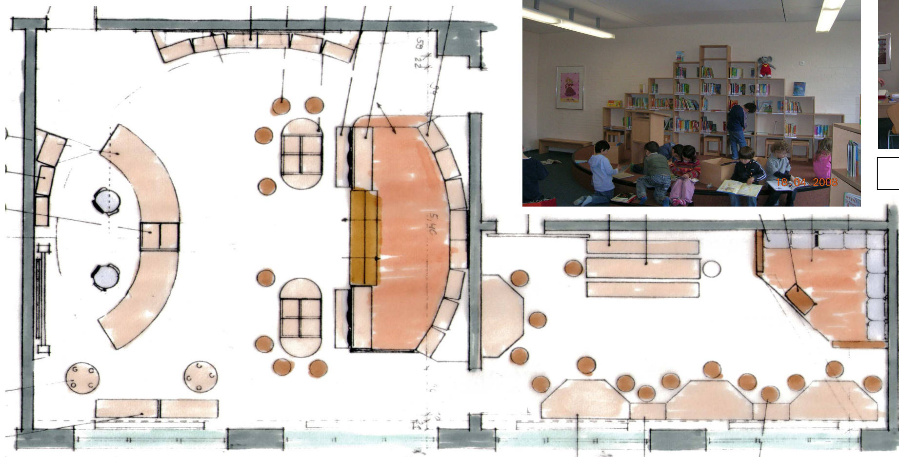
Entwurfsplanung der Schülerbücherei mit angrenzendem Arbeitsraum. Umgesetzt wurde im ersten Schritt der vordere Raum mit einigen Änderungen im Detail
